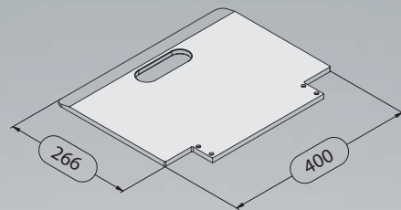
Pelle 400 x 266 mm
