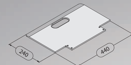
Pelle 440 x 240 mm
