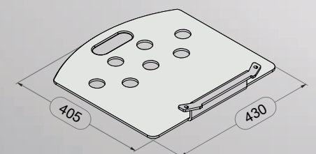
Pelle avec point de fixation 430 x 405 mm
