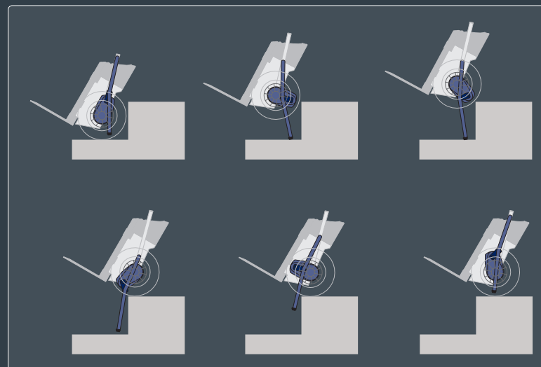
La cinématique ascensionnelle brevetée franchit en toute sécurité marche après marche
