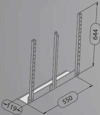
Standard 12 cm - montants allongés 550 x 119 x 644 mm
