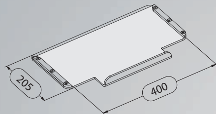
Pelle pour caisses de boissons à suspendre 400 x 205 mm
