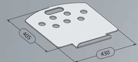
Pelle à rideaux 430 x 405 mm
