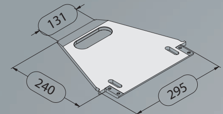
Pelle en V 295 x 240 mm
